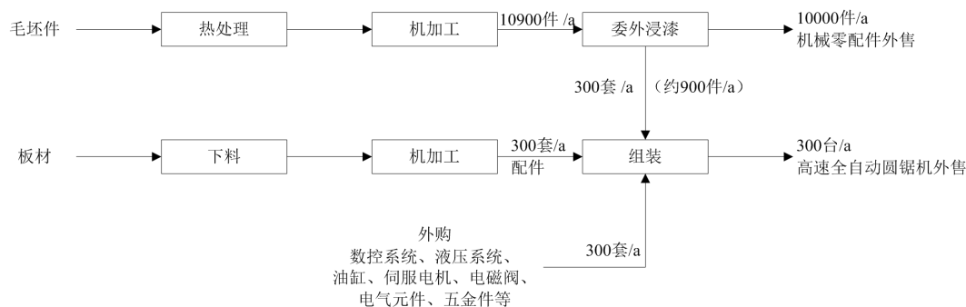
图 9.1-1 生产流水线工艺图
