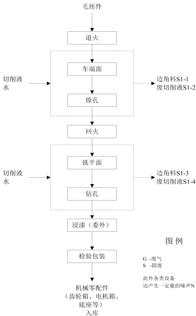
图 3.5-1 机械零配件生产工艺流程及产污节点图
