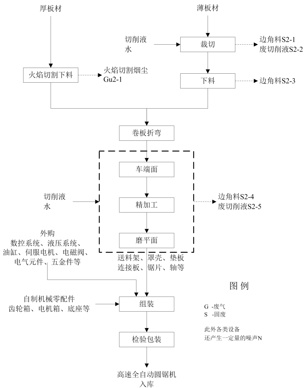
图 3.5-2 高速全自动圆锯机生产工艺流程及产污节点图
