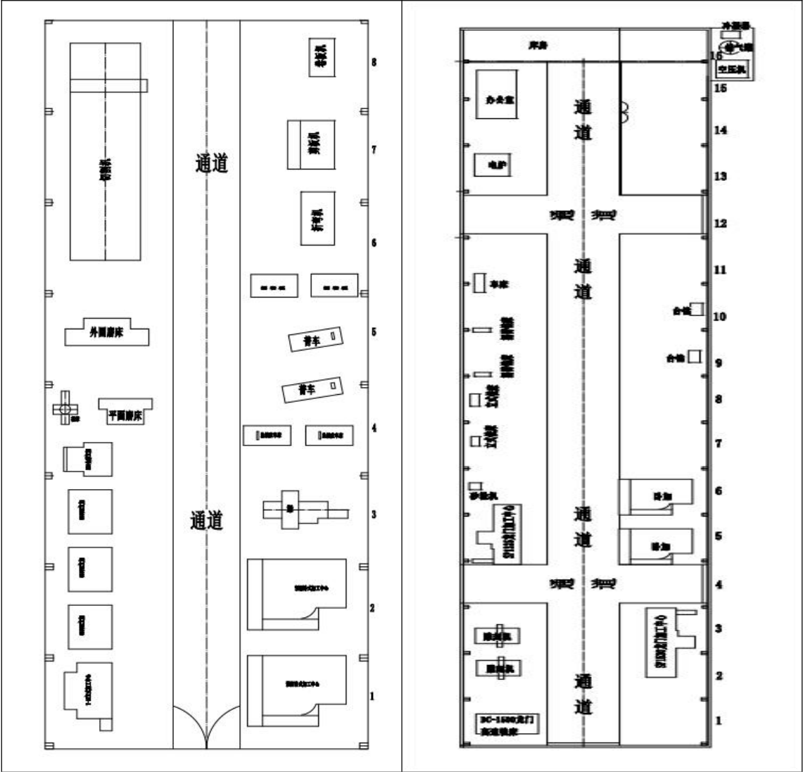
图 3.2-1 设备现场布置图
