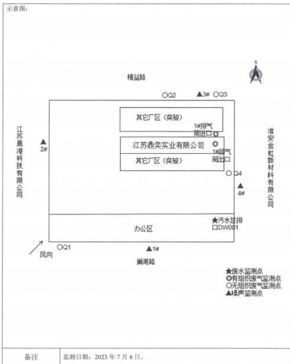
图 7.5-2 项目验收监测点位 (2023 年 7 月 6 日)
