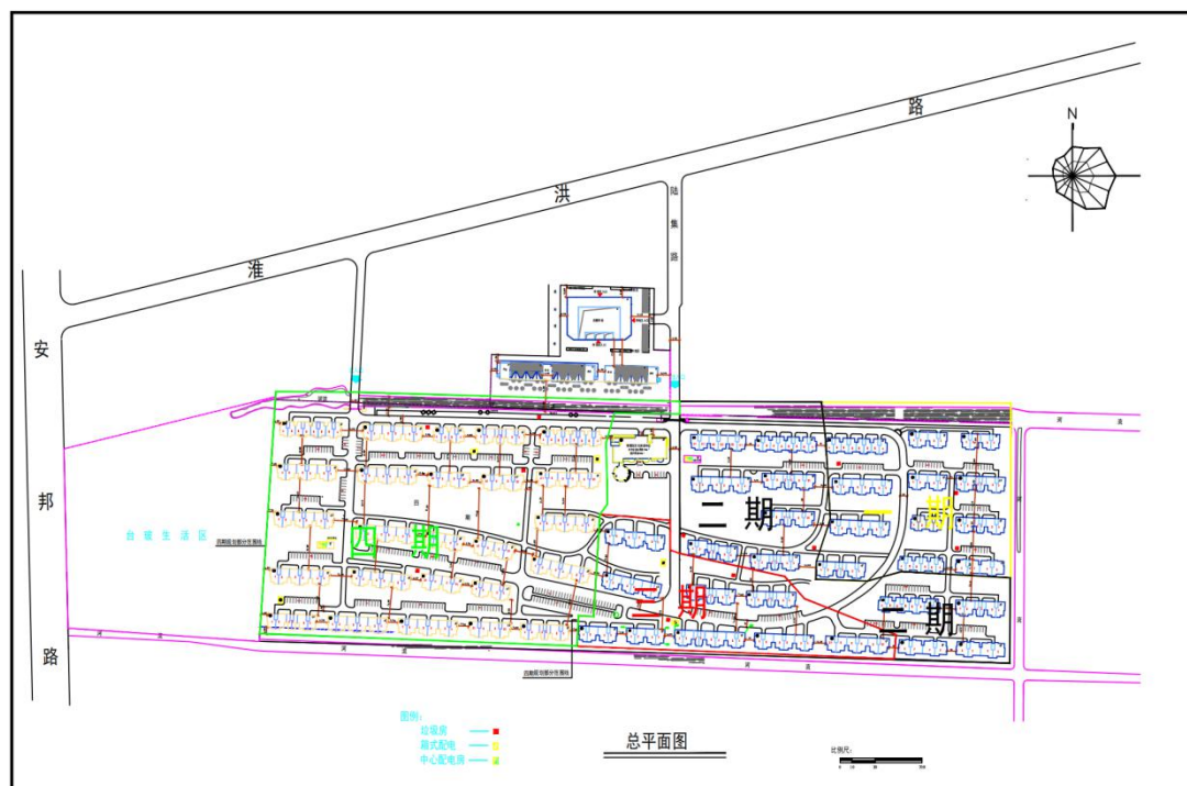
图 3.1-3 盐化工安置小区平面布置图
